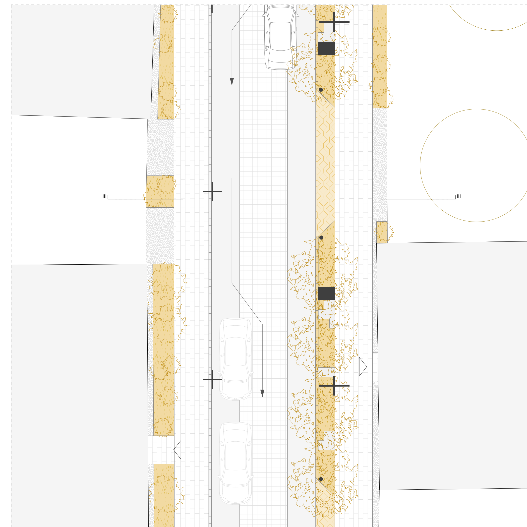
LOIGE III - III KOOS PLAANIFRAGMENTIDGA (KITSENDATUD LIIKLUSEGA TÄNAVALOIK) M 1:100
