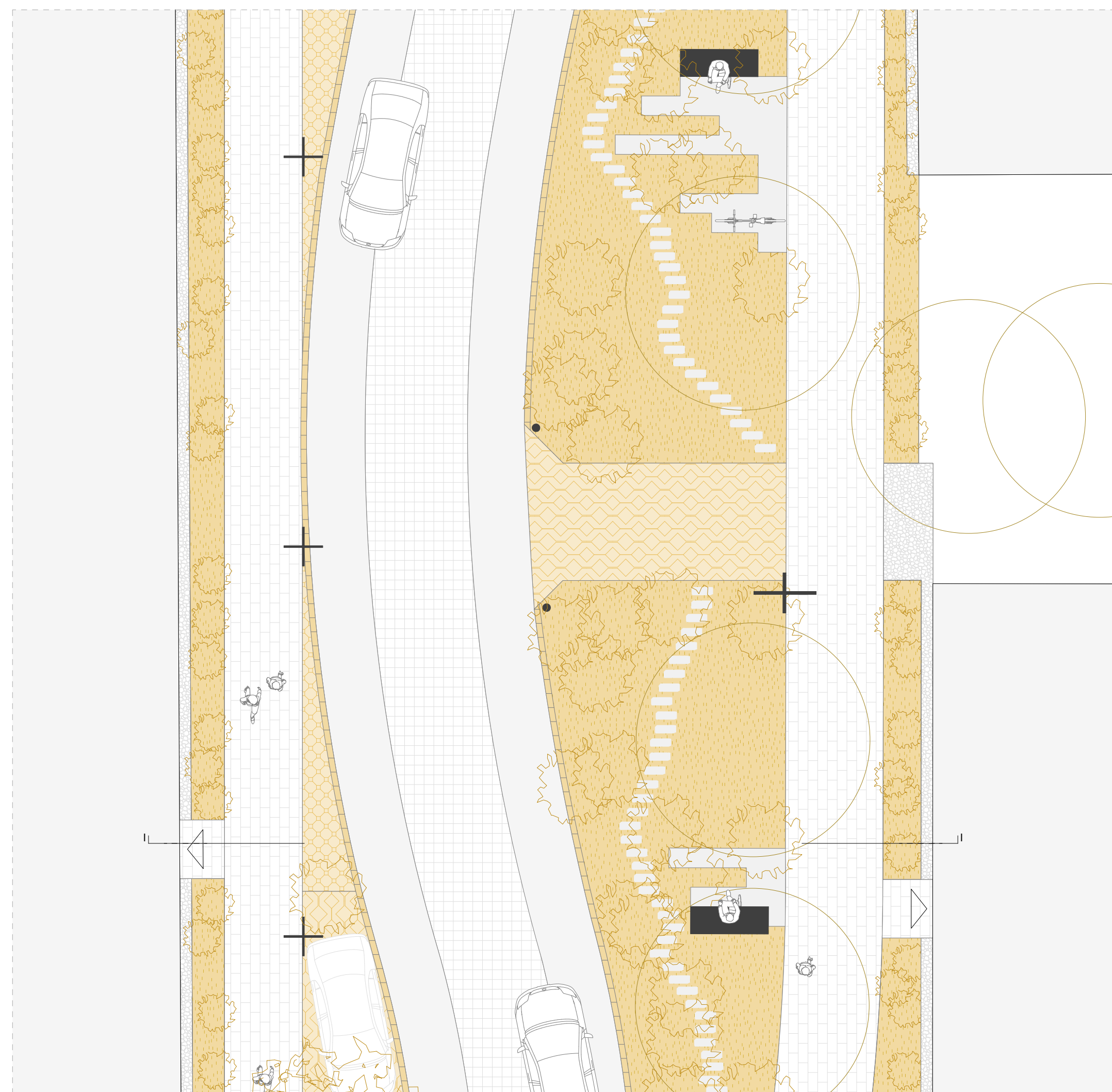
LOIGE I - I KOOS PLAANIFRAGMENTIDGA (KAHESUUNALINE TÄNAVALOIK) M 1:100
