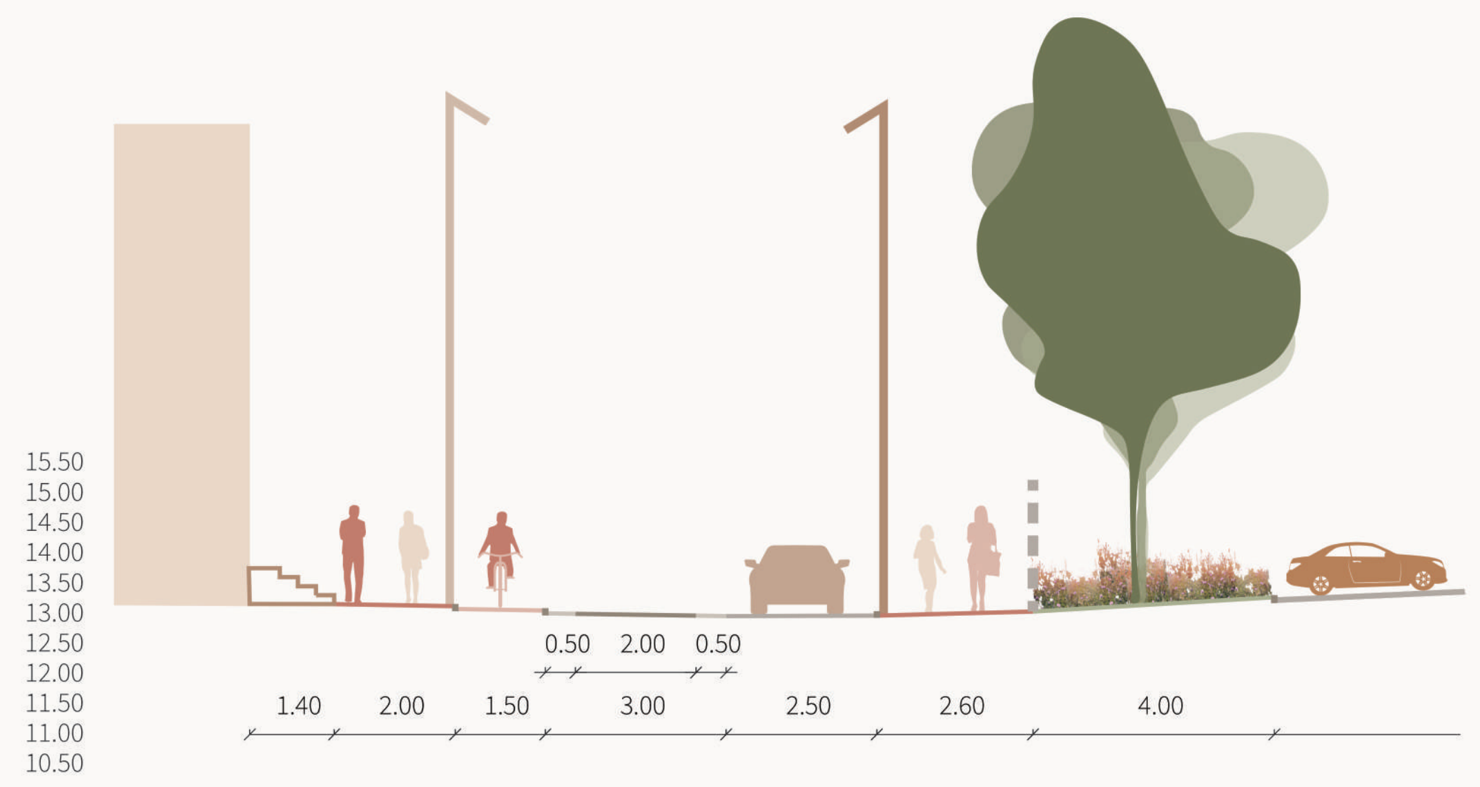
lõige 5-5
