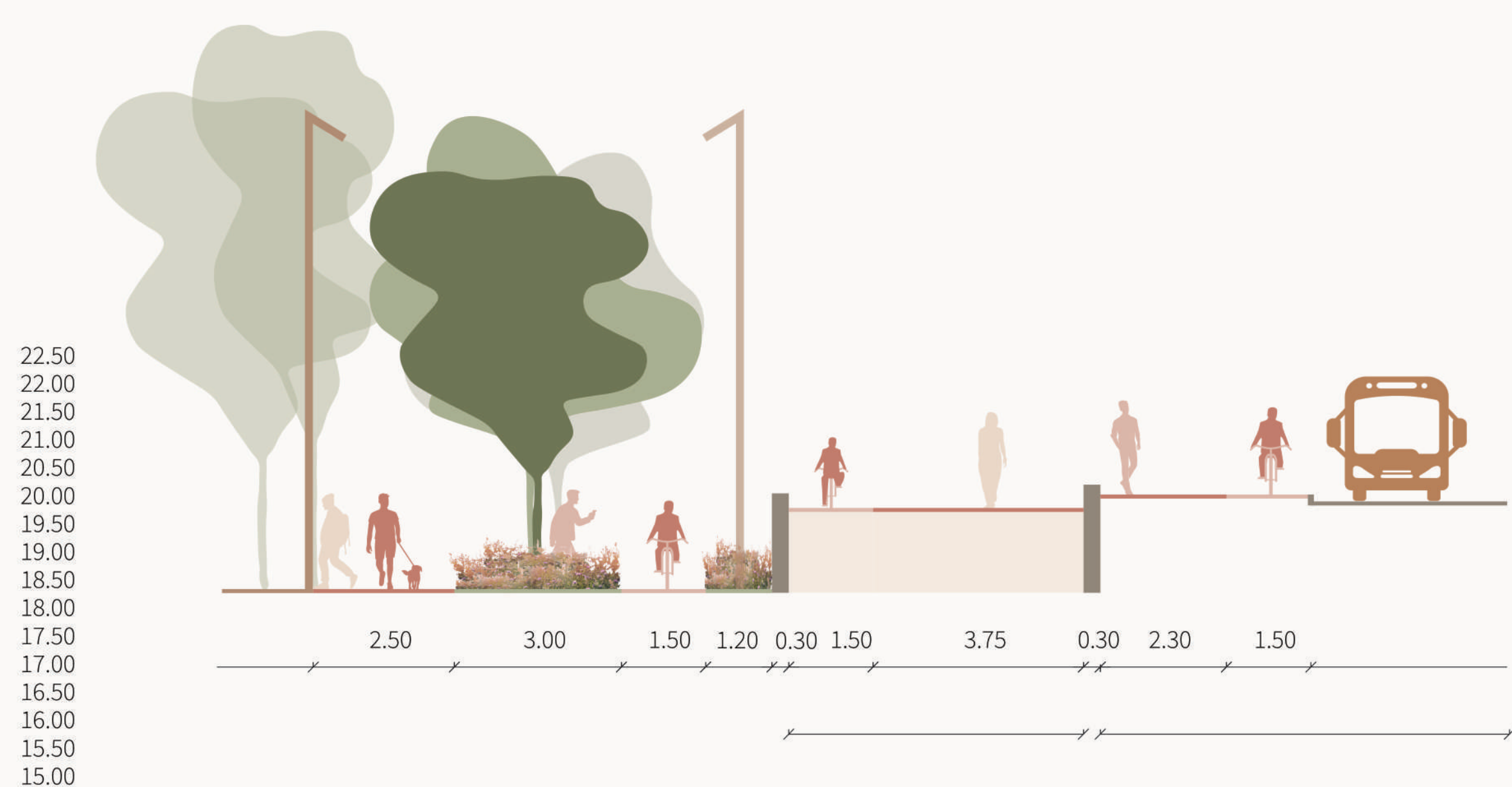
lõige 8-8
